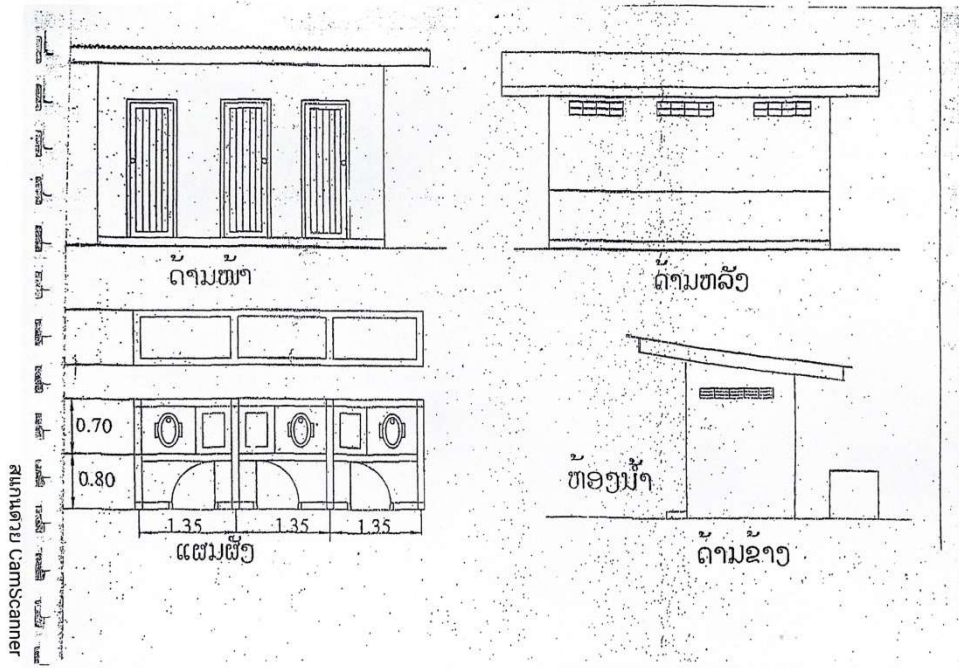
Voici le plan du bâtiment de 3 toilettes latrines
